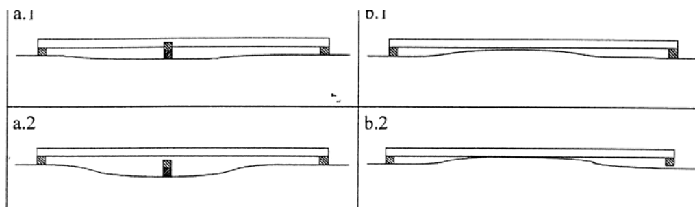
Figuur 1; Vlakheidsmeting
